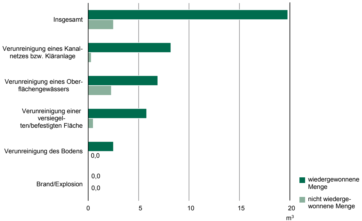
Abb. 1 Freigesetzte Menge 1) 2) durch Unfälle beim Umgang mit wassergefährdenden Stoffen in Sachsen 2017 nach Unfallfolgen
