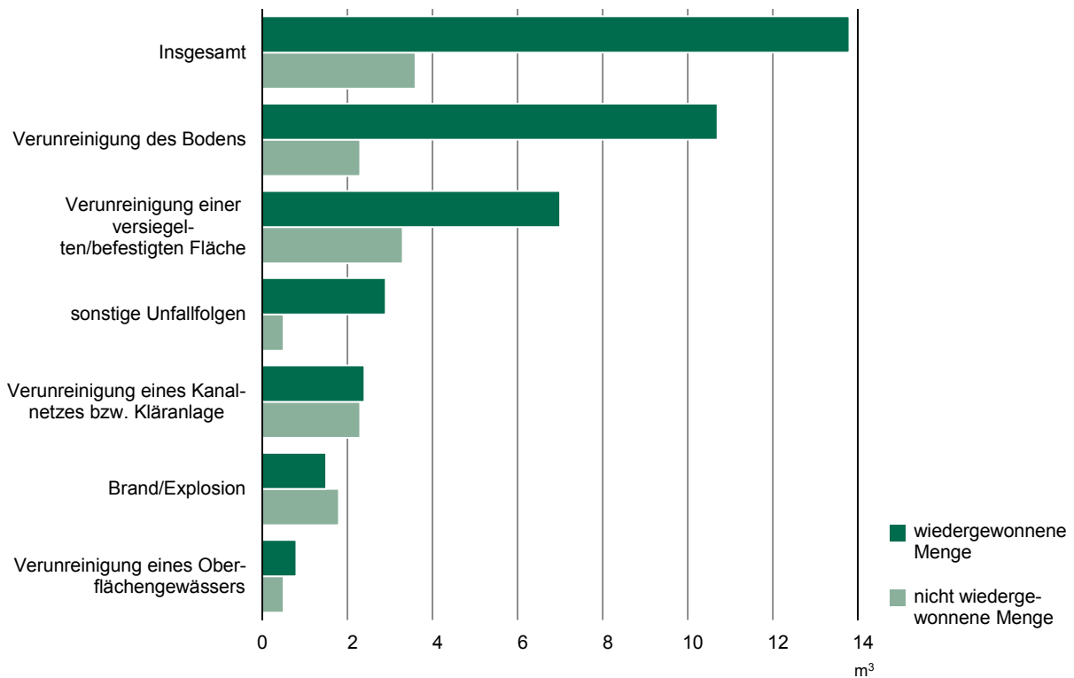
Abb. 2 Freigesetzte Menge 1) durch Unfälle bei der Beförderung wassergefährdender Stoffe in Sachsen 2017 nach Unfallfolgen
