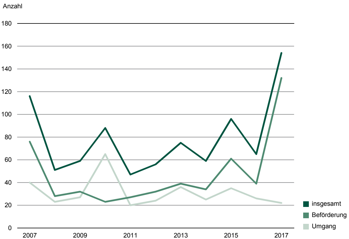
Abb. 4 Unfälle bei der Beförderung und im Umgang mit wassergefährdenden Stoffen 2007 bis 2017
