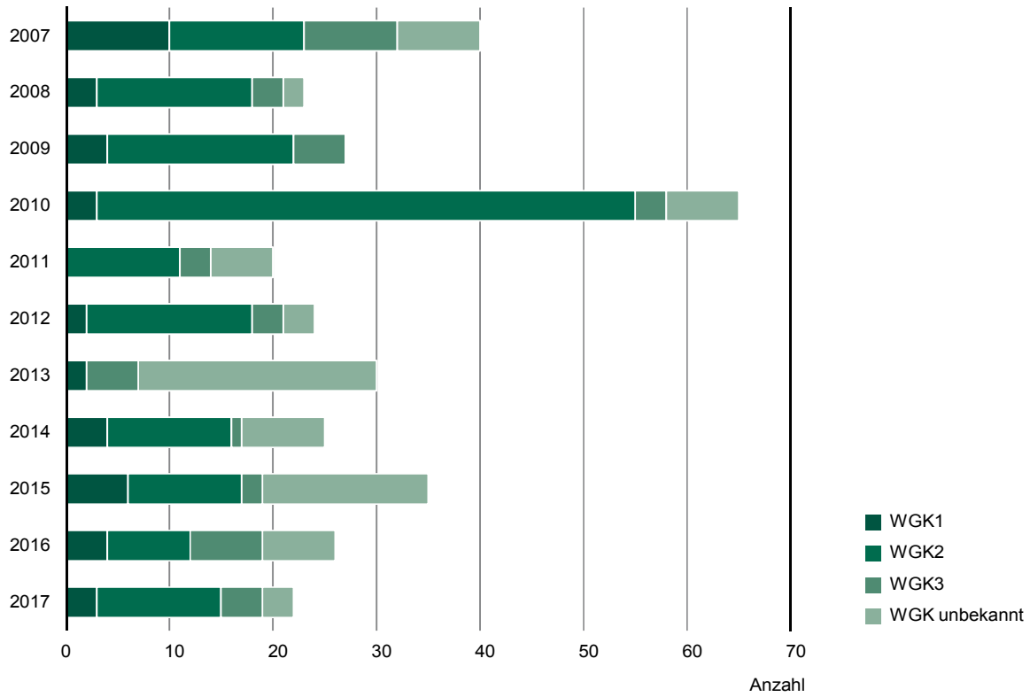
Abb. 5 Anzahl der Unfälle beim Umgang mit wassergefährdenden Stoffen 2007 bis 2017 nach Wassergefährdungsklassen
