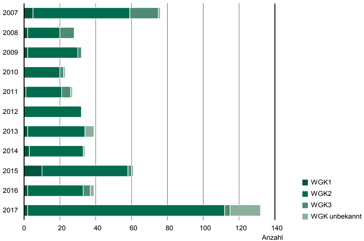
Abb. 6 Anzahl der Unfälle bei der Beförderung mit wassergefährdenden Stoffen 2007 bis 2017 nach Wassergefährdungsklassen
