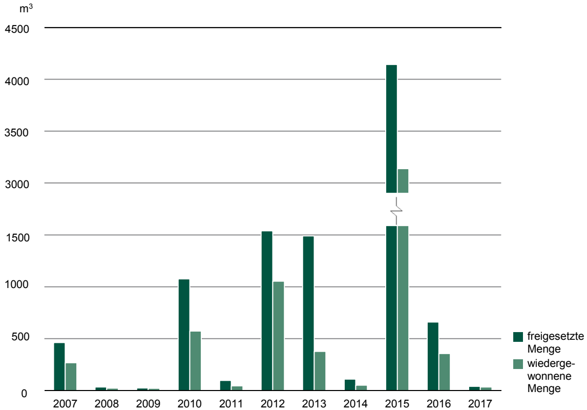
Abb. 3 Freigesetzte und wiedergewonnene Mengen bei Unfällen mit wassergefährdenden Stoffen 2007 bis 2017
