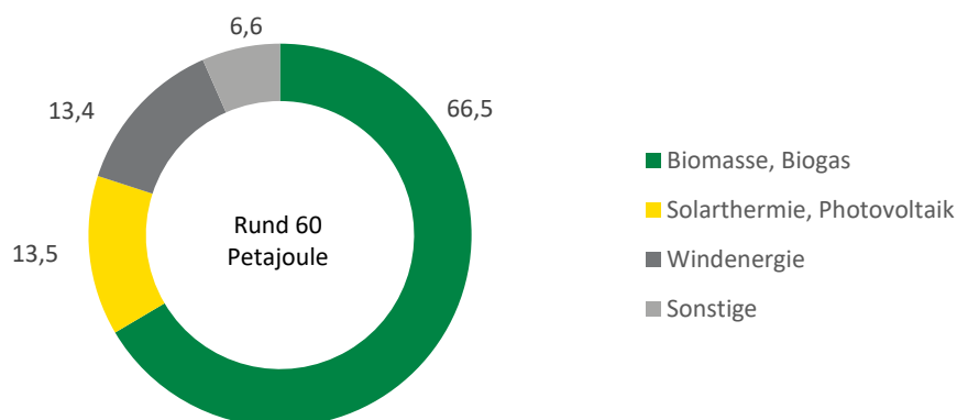
Primärenergieverbrauch Erneuerbarer Energieträger in Sachsen 2019 in Prozent
