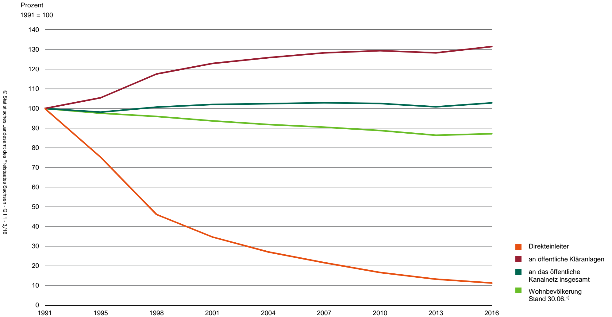
Abb. 16 An die öffentliche Abwasserentsorgung angeschlossene Einwohner im Freistaat Sachsen 1991 bis 2016
